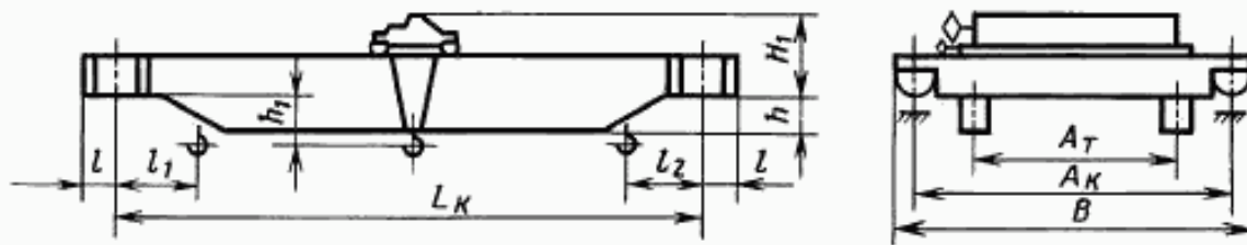
Двухбалочные краны
